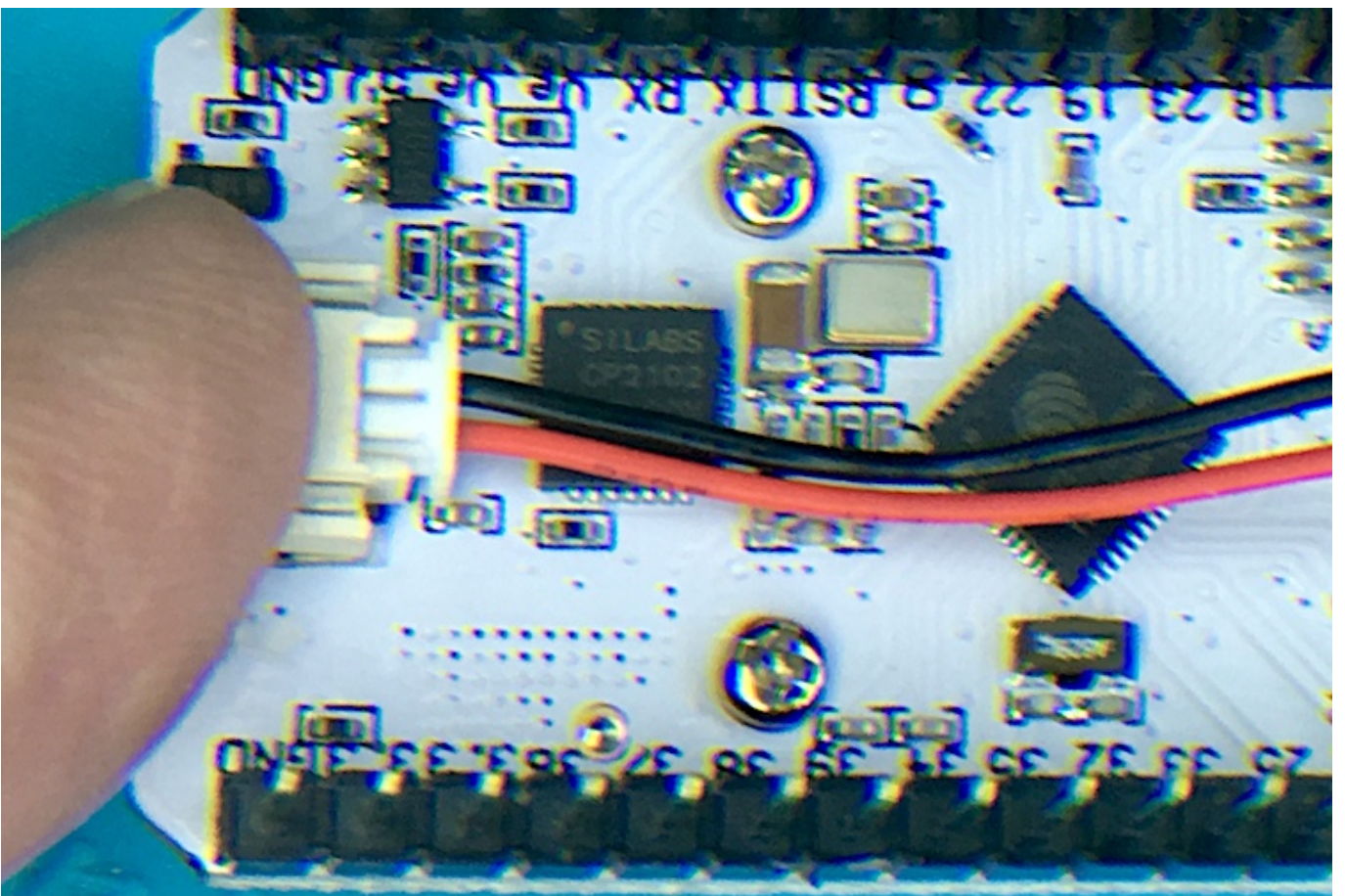
Befestigen des Anschlusskabels
