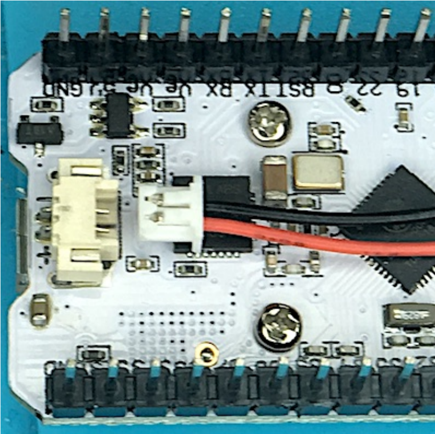
Ausrichtung des Anschlusskabels
