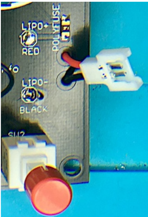
Anschlusskabel montiert für Akku unter Heltec Modul
