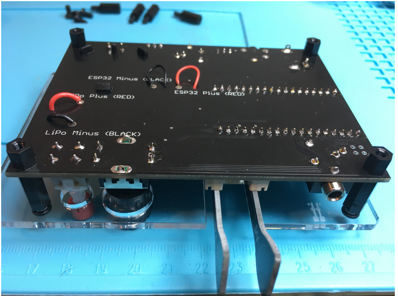
Ansicht Platinenunterseite
